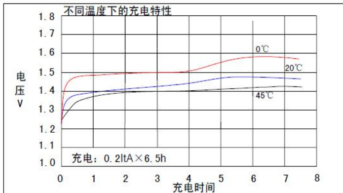
特征曲线
